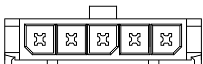
5-CKT
